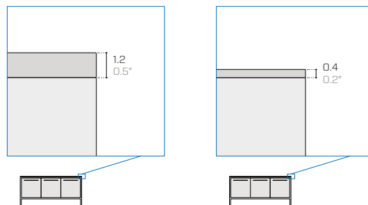
Top made of Fenix Top in Fenix Arbeitsplatte aus Fenix
